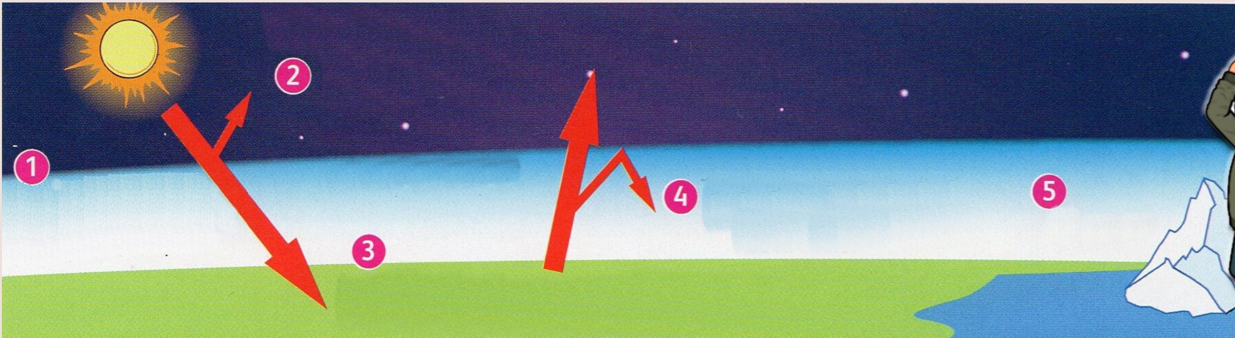
L'effet de serre sur la planète.
